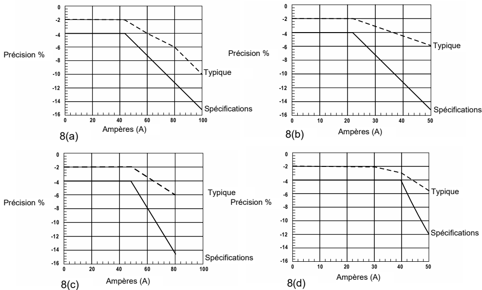
Figure 8(a - d): Linéarité pour Signal DC, gamme 0.1 V/A, typique
