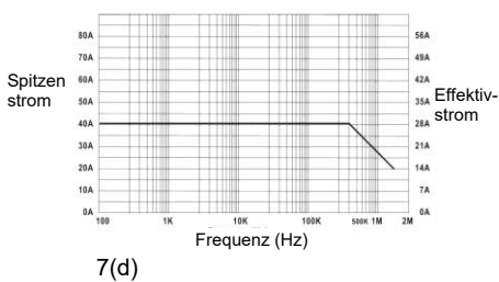
Abbildung 7(a – d): Maximaler Strom gegen Frequenz
