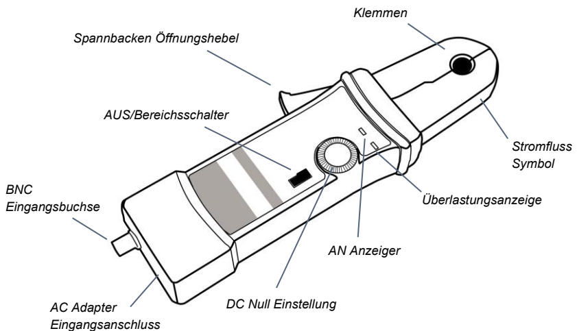
Abbildung 1: zeigt die Bedienelemente und Anzeige an der Stromzange
