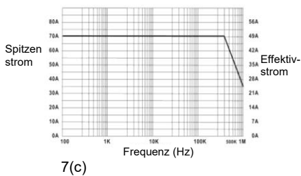
Abbildung 7(a – d): Maximaler Strom gegen Frequenz
