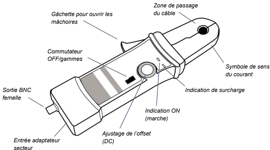
Figure 1: face avant de la pince
