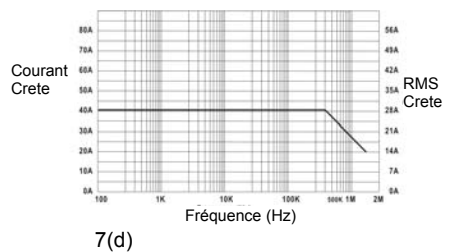
Figure 7(a – d): Courbe Courant crete/Fréquence
